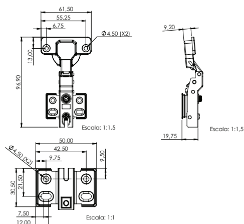
Dobradiça Calço Fixo 35mm Curva Soft Closing
