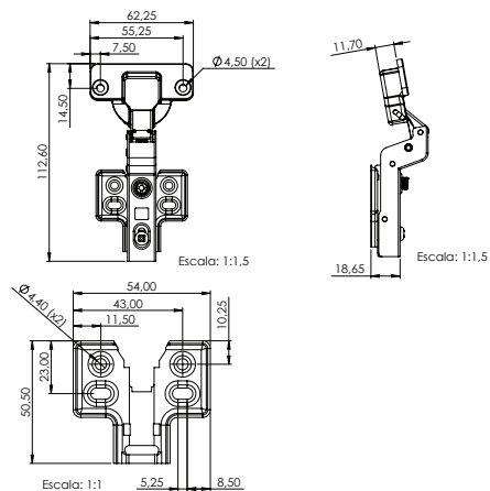
Dobradiça 35mm Inox Super Curva com Pistão Calço Click
