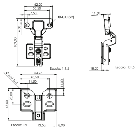
Dobradiça 35mm Inox Super Curva com Pistão Calço Fixo
