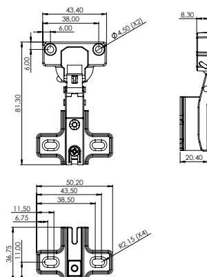
Calço 12
