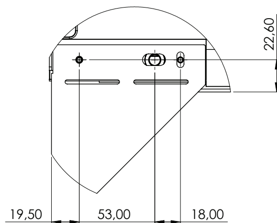
DETALHE B
