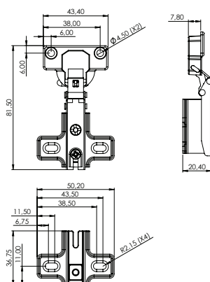
Calço 12
