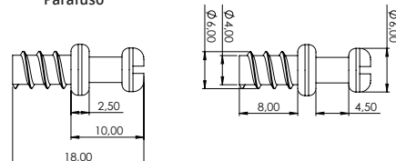
Parafuso
