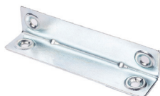
002.02.014 Cantoneira Metálica 80x18x18mm para Gaveta
